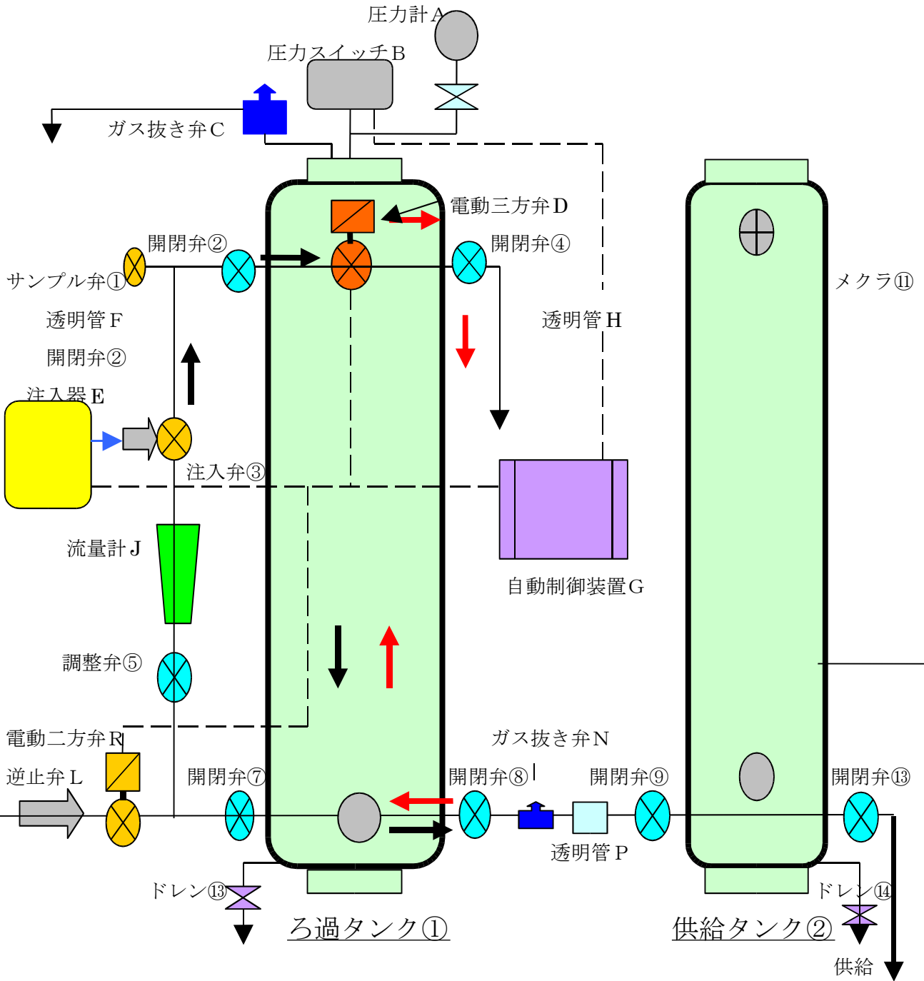
[井戸ポンプが圧カスイッチ制御の設置例]
